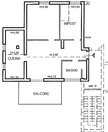
PIANO SECONDO (SOTTOTETTO)
