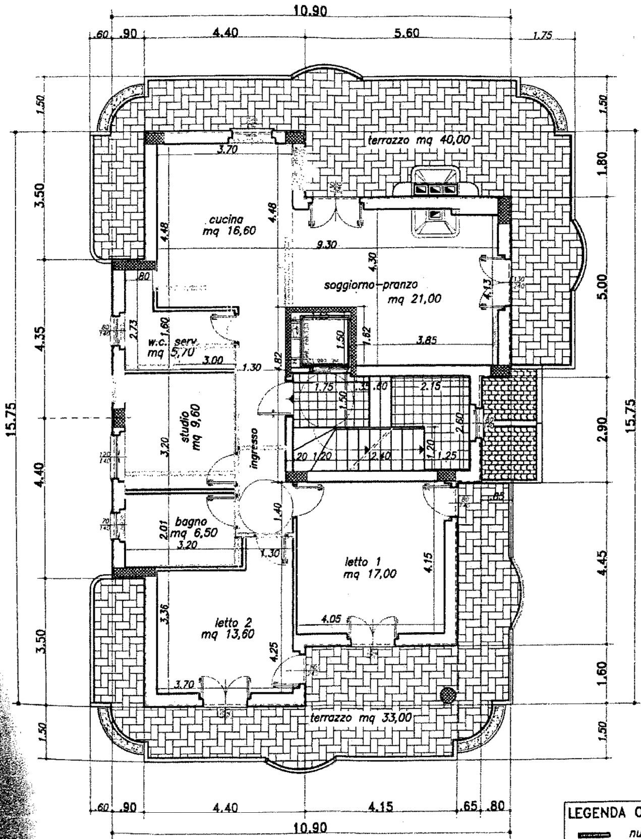
PIANTA PRIMO PIANO -Interno 1-
